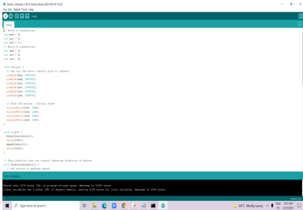
Fig 10.1: Arduino IDE
